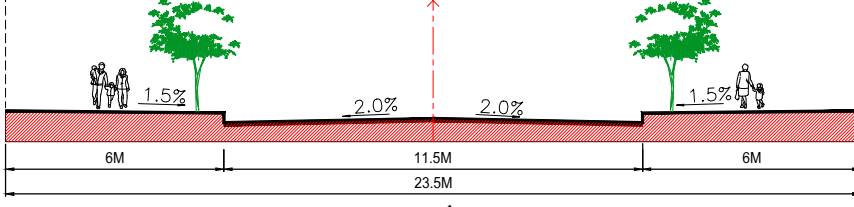
MẶT CẮT 5-5
