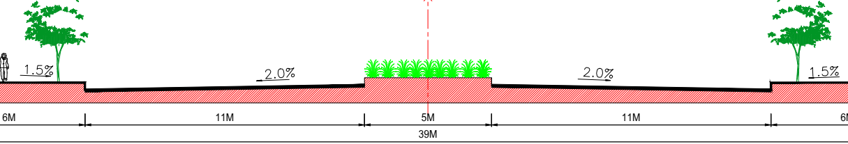
MẶT CẮT 3-3
