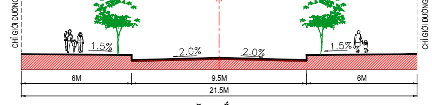
MẶT CẮT 6-6
