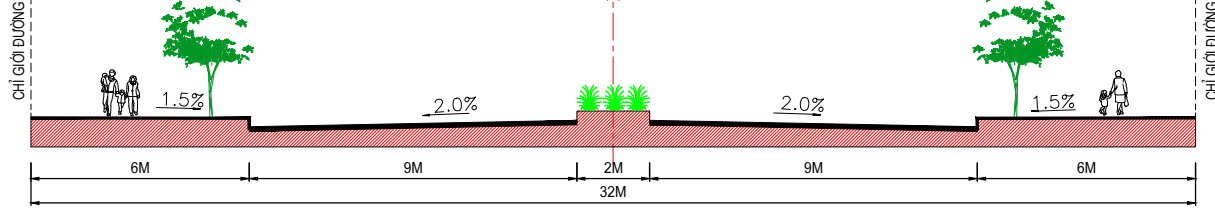
MẶT CẮT 2-2
