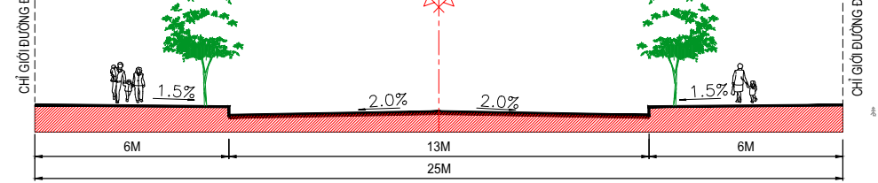
MẶT CẮT 7-7
