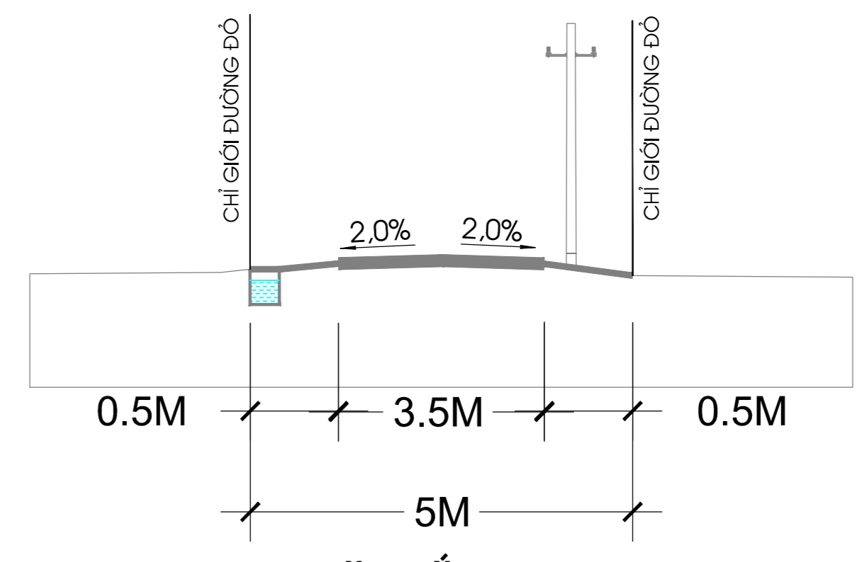
MẶT CẮT 4-4 (ĐƯỜNG NỘI ĐỒNG)
