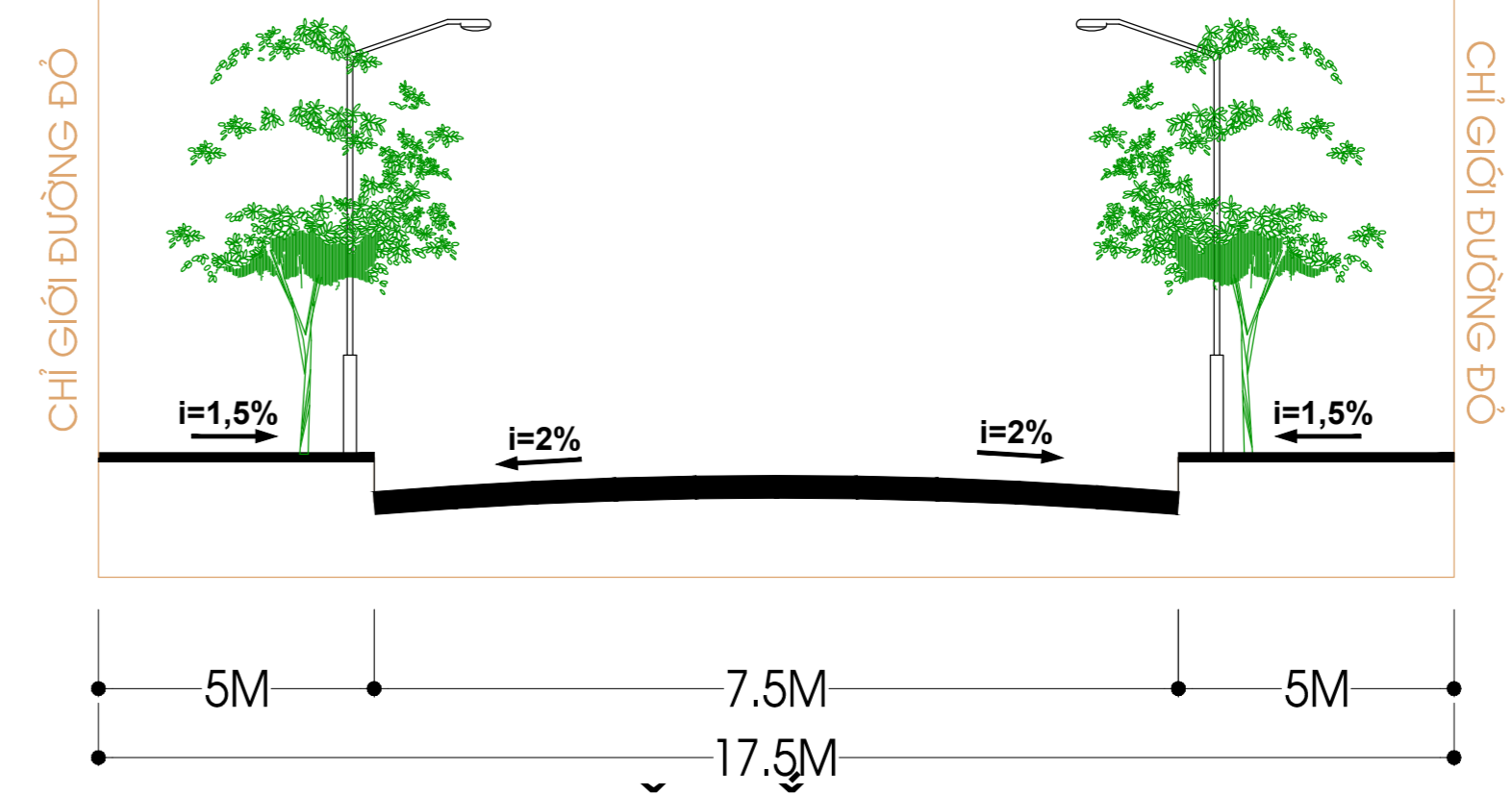
MẶT CẮT 1-1 (TUYẾN ĐƯỜNG LIÊN XÃ)
